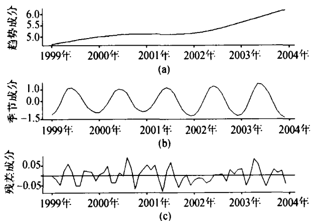
图 2 DHR 模型分离出各成分 (a) 趋势成分; (b) 季节成分; (c) 残差成分
