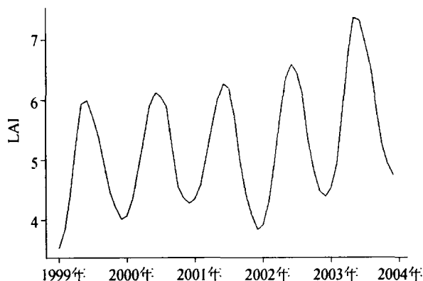
图 1 LAI 时间序列(1999—2004 年)
