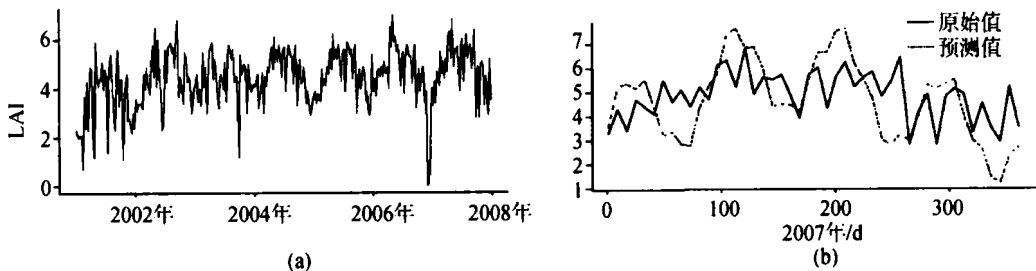
图 5 常绿林类像元预测结果 (a) LAI 原始时间序列 2001—2007 年; (b) 该像元点 2007 预测结果与原始数据比较
