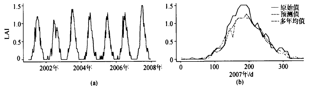
图 4 像元点预测结果 (a) 像元 LAI 原始时间序列 2001—2007 年; (b) 2007 年该像元点预测结果与原始序列比较
